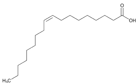
Oleic acid
